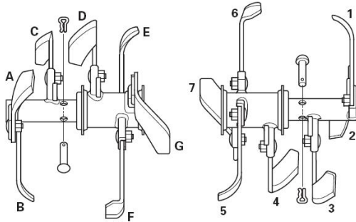
Oikea teräpakka R (kuvaus oikealta)
